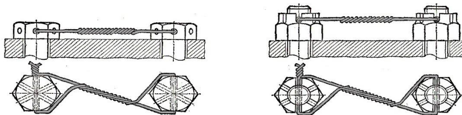
Рис. 18. Пример контровки резьбового соединения.
