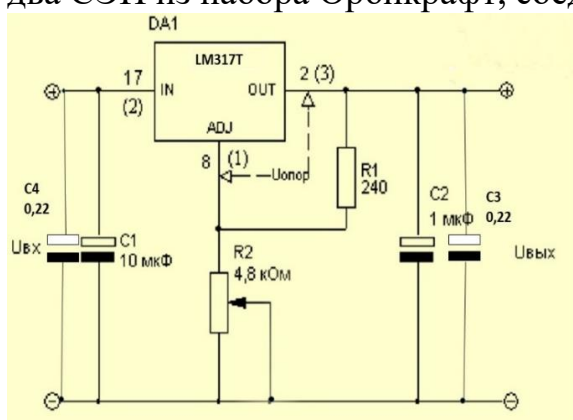
Рис. 15. Стабилизатор напряжения
